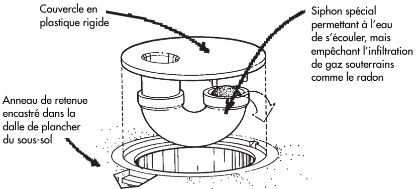
Figure 18. Siphon destiné aux nouveaux avaloirs de sol
