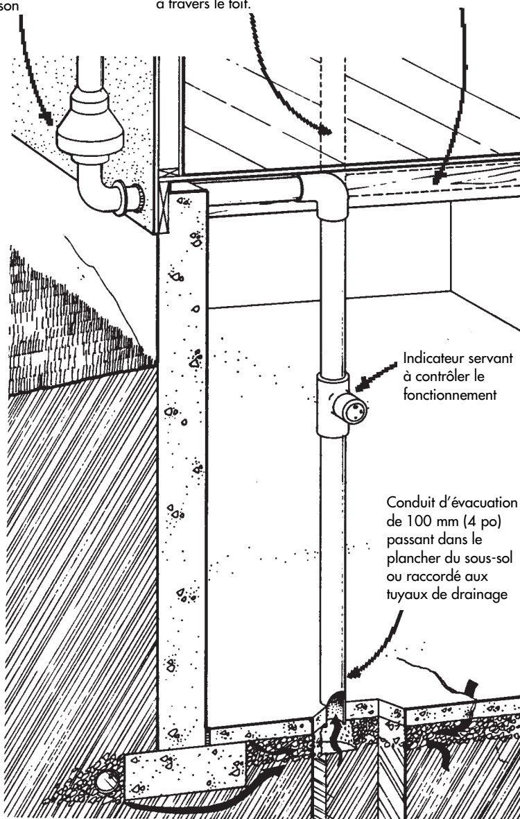
Figure 11. Installation de dépressurisation du sol
