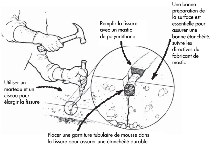
Figure 12. Obturation des fissures dans les murs de fondation et les planchers
