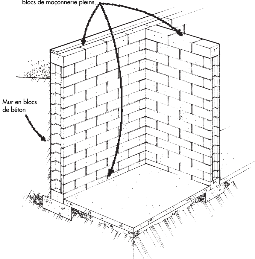
Figure 19. Élimination des cavités au haut et au bas des nouveaux murs de fondation en blocs de béton.
