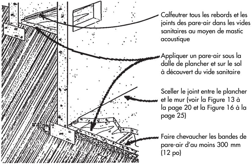
Figure 17. Pare-air de polyéthylène pour vide sanitaire et dalle de plancher de sous-sol
