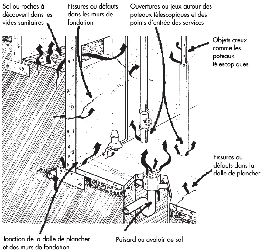
Figure 2. Points d'entrée habituels du radon dans les murs de fondation et les planchers en béton coulé
