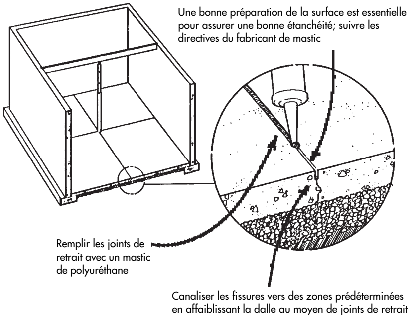
Figure 15. Joints de retrait pour les nouvelles dalles de plancher en béton
