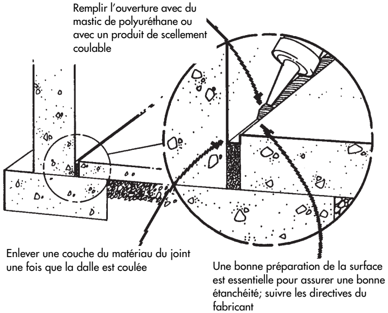
Figure 16. Obturer la jonction entre le mur de fondation et le plancher du sous-sol dans les constructions neuves
