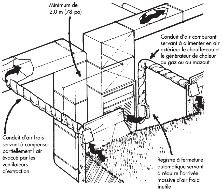
Figure 20. Réduction des différences de pression au moyen de conduits d'air frais et d'air comburant
