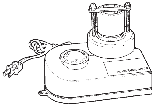
Figure 6. Détecteur alpha de type actif
