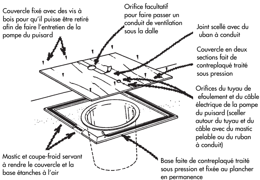
Figure 8. Scellement des puisards ouverts
